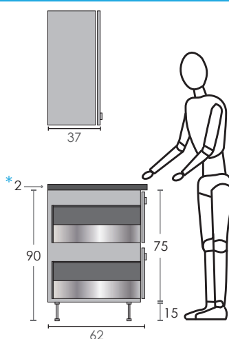
Zone de travail – hauteur 92
