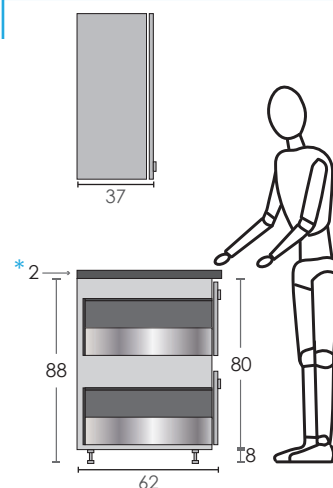
Zone de travail – hauteur 90
